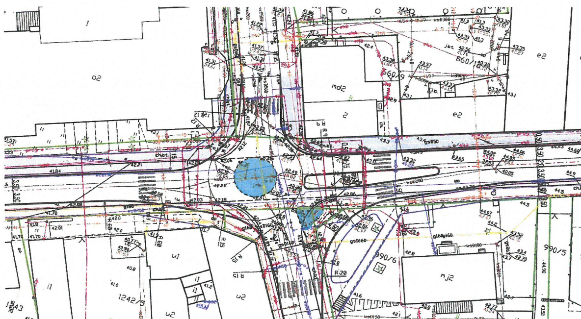
Rysunek: Koncepcja przebudowy skrzyżowania ul. Wojska Polskiego z ul. Sienkiewicza i ul. Mickiewicza, źródło: własne
