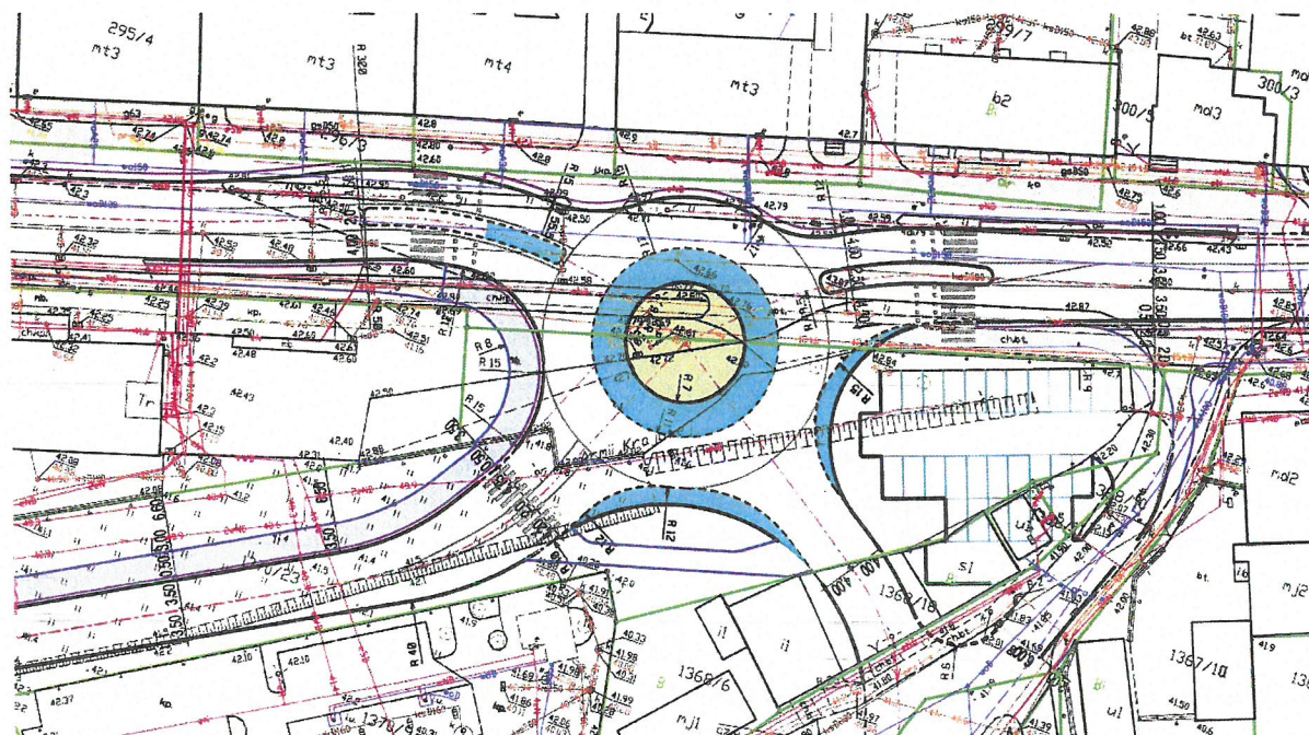
Rysunek: Koncepcja przebudowy skrzyżowania ul. Wojska Polskiego z ul. Armii Krajowej, źródło: własne
